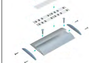
Perfil - R Difusor - Basic
